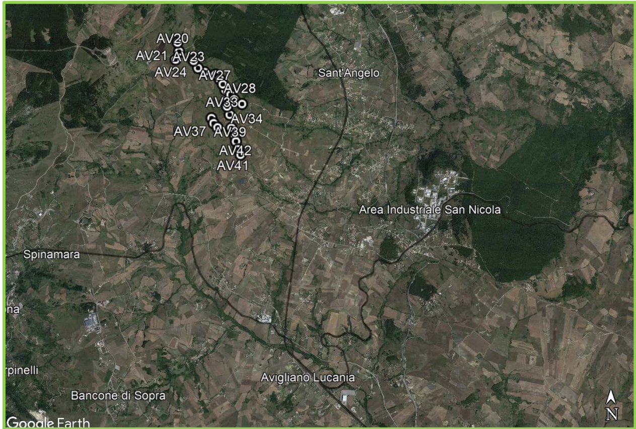
Figura 1 - Parchi Eolici "AVIGLIANO I e AVIGLIANO II CV".
