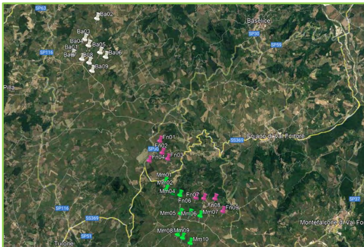
Figura 1 - Parco Eolico "FOIANO-BASELICE-MOLINARA".
