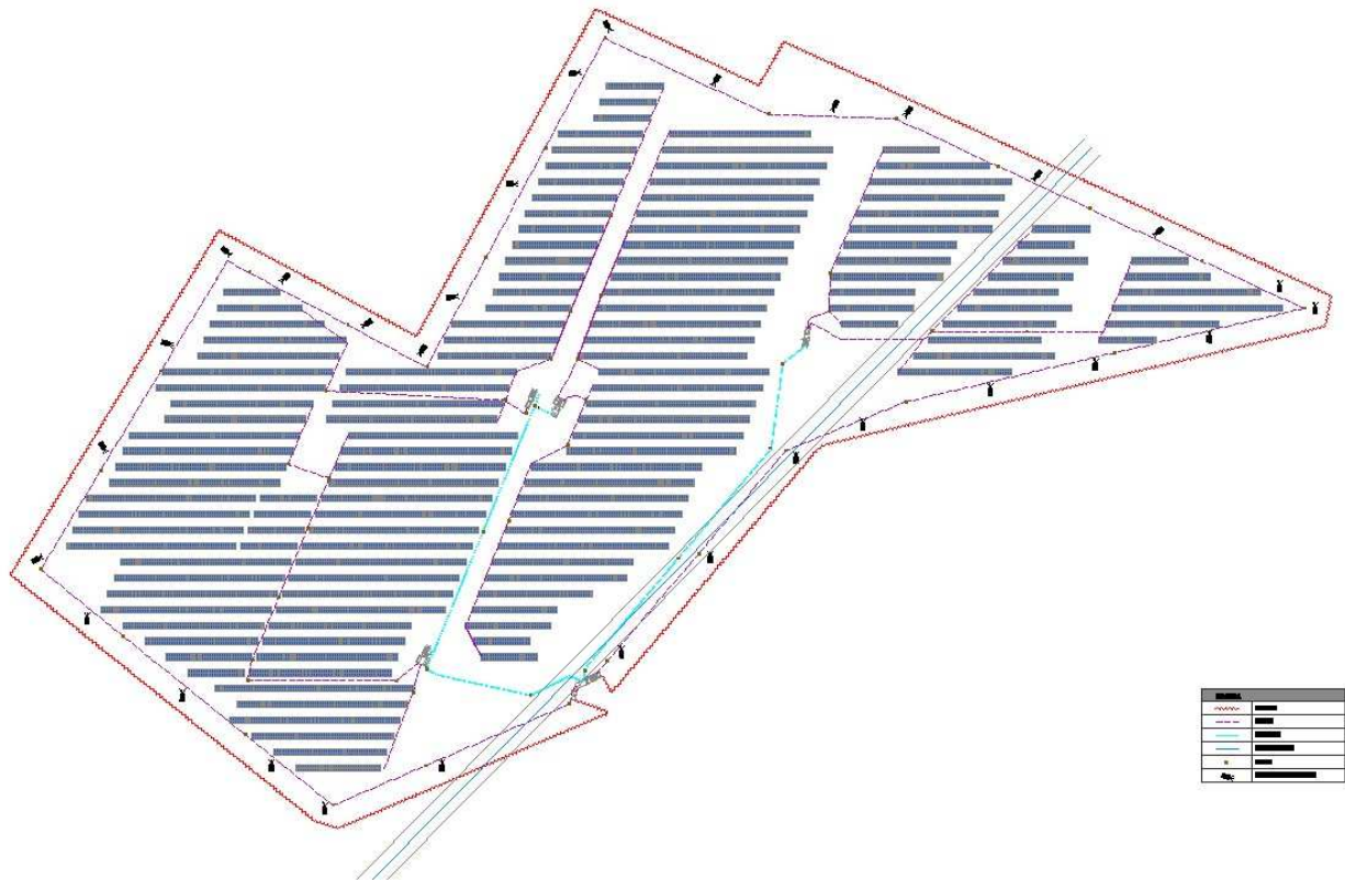
Figura 2: Planimetria aerea Tav.01
