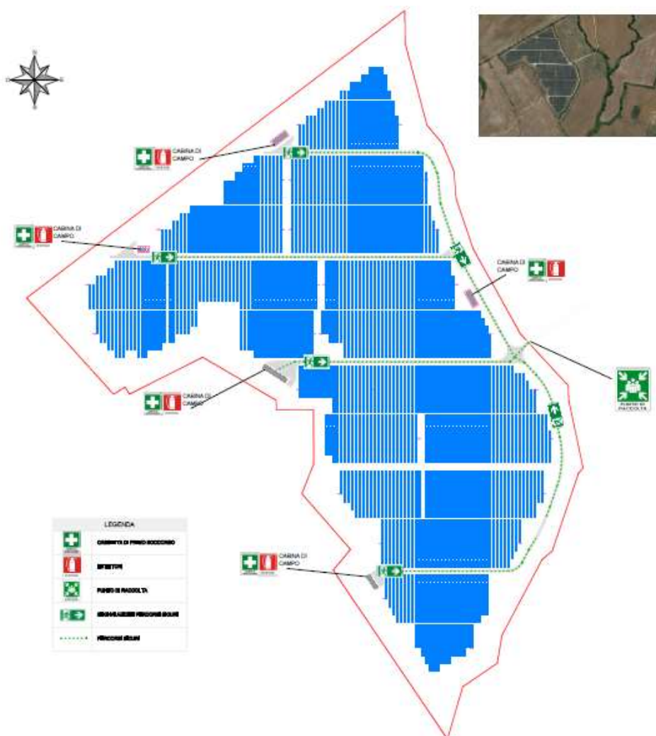
Figura 2 Planimetria d'impianto
